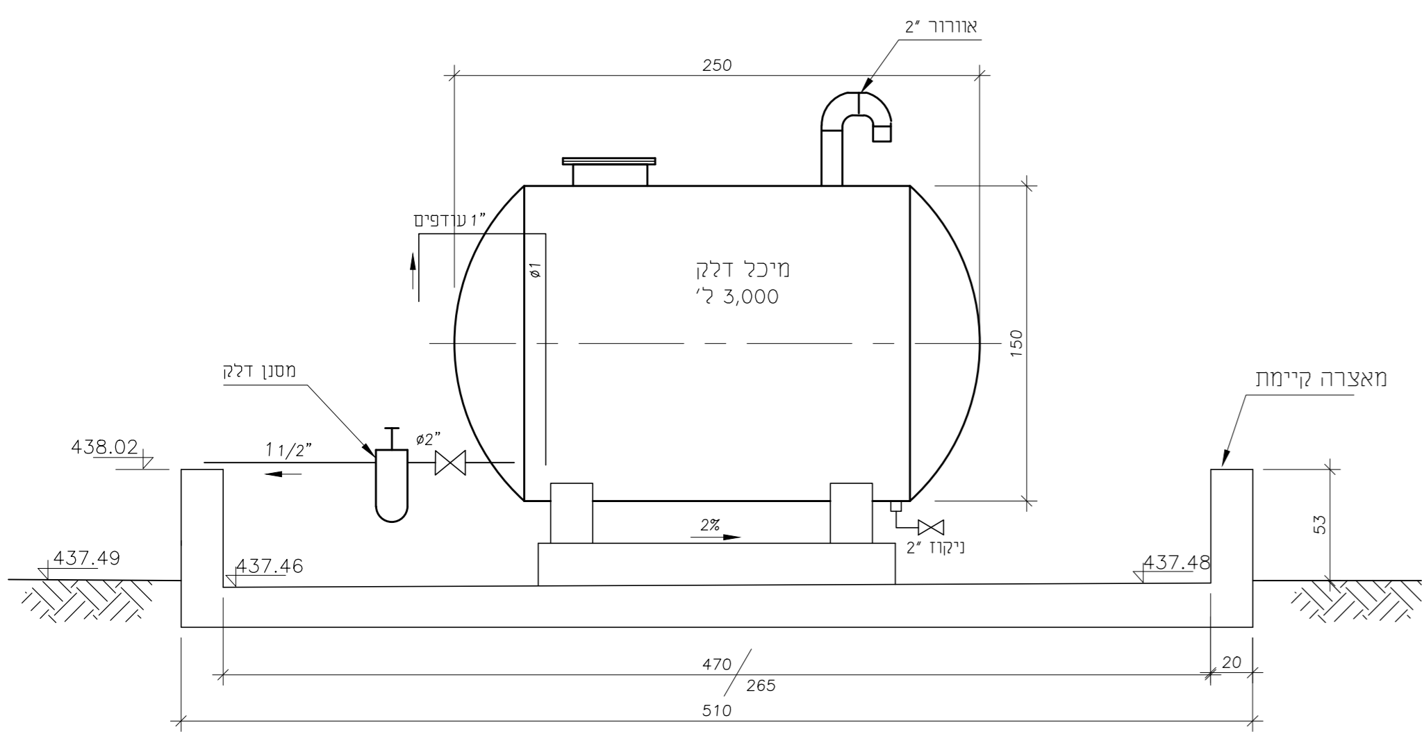
חתך הי - הי קו"מ 125
